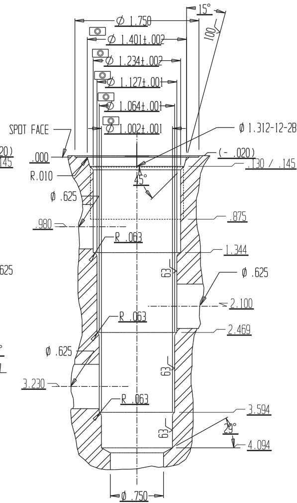
CAVITY 5053-16-4
